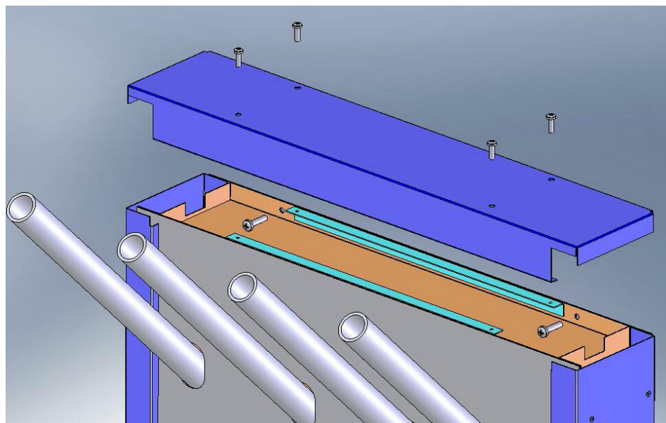
Рис. 7 Схема крепления сушильной панели к стене помещения
